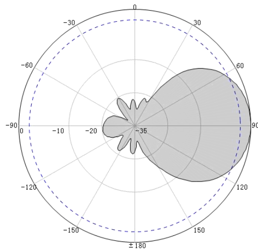
600MHz-Vertical Pattern
