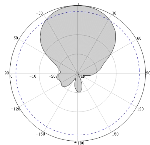
600MHz- Horizontal Pattern
